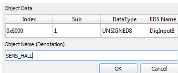
Dialog zum Umbenennen eines Objekts
