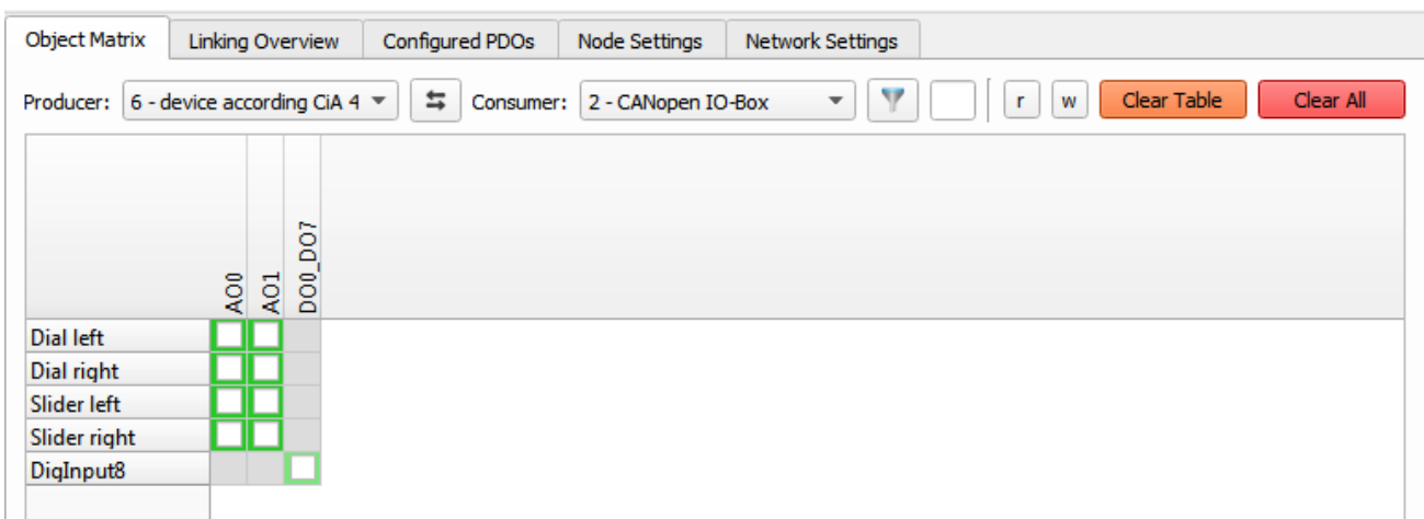
Object Matrix mit verknüpften Objekten
